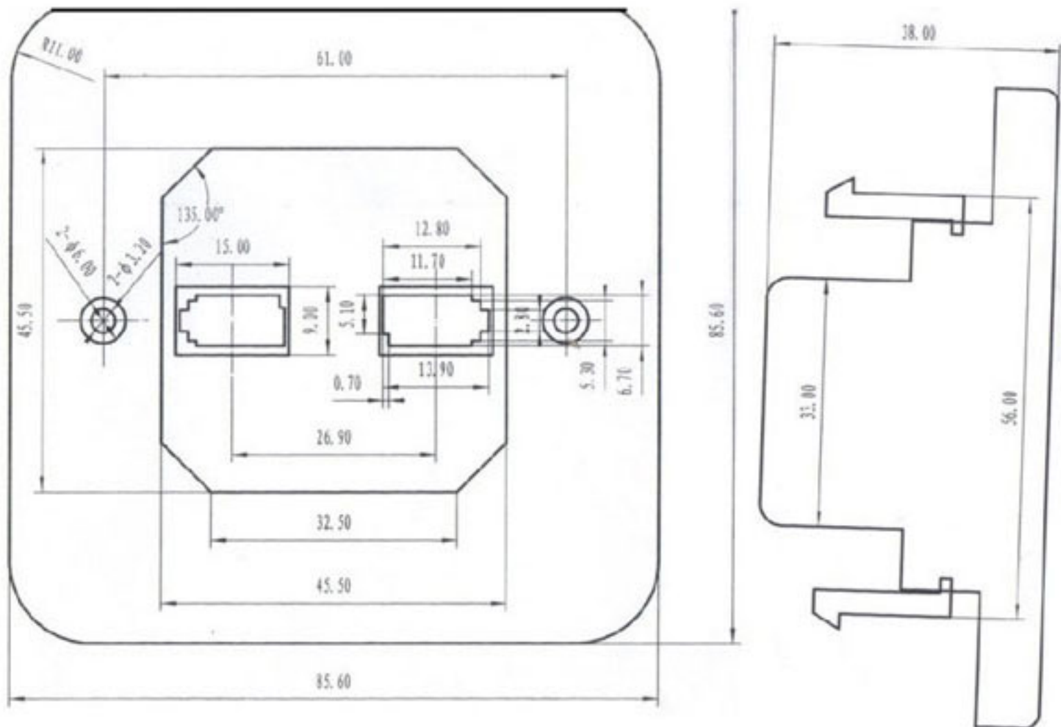
一般公差
